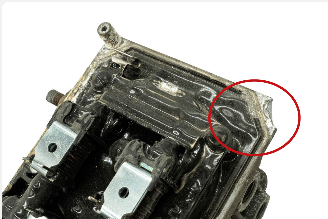
Uszkodzone mocowanie elektroniki w korpusie
