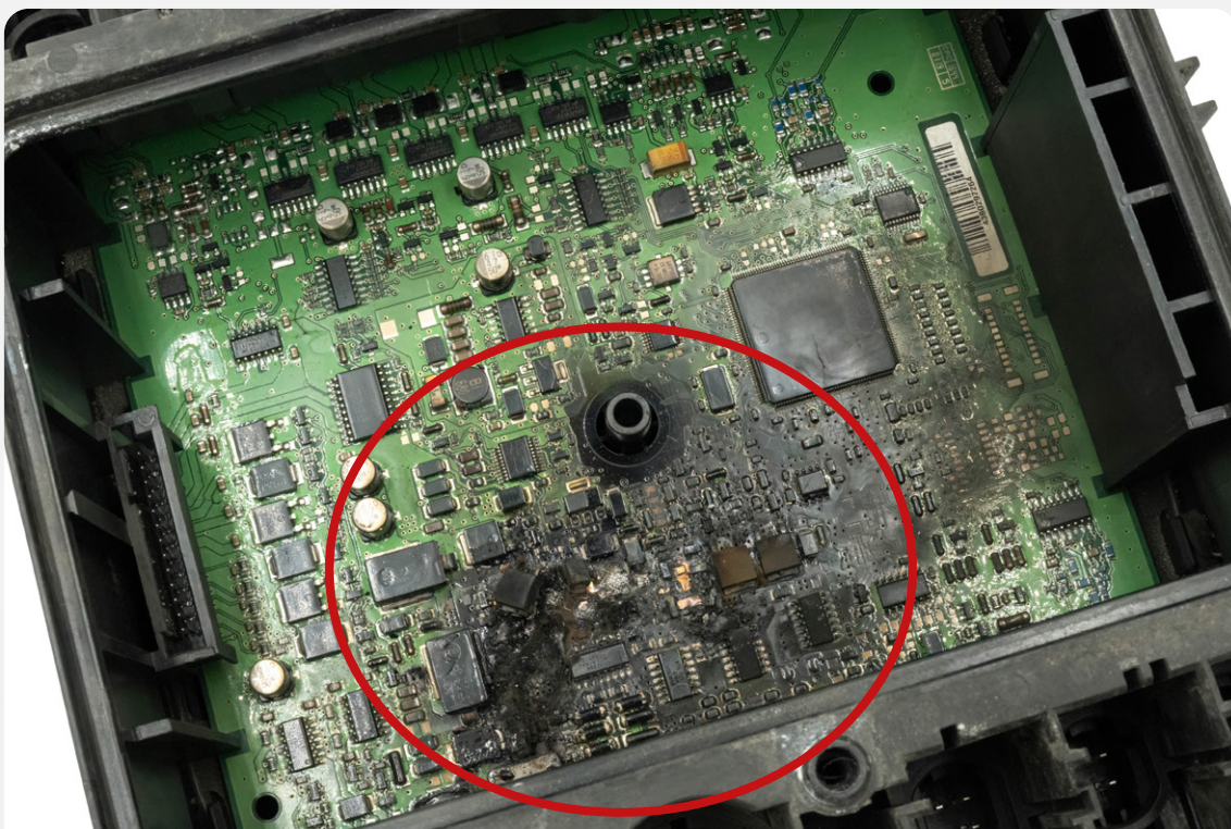
Spalona płyta elektroniczna
