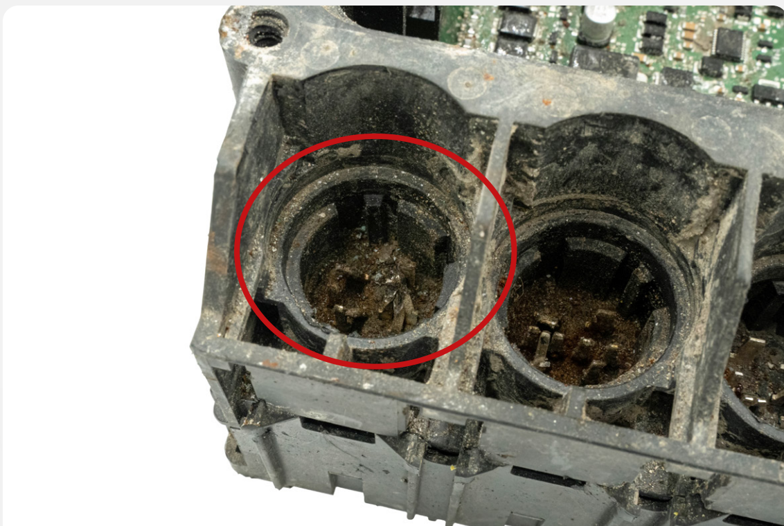
Uszkodzone gniazdo elektroniczne
